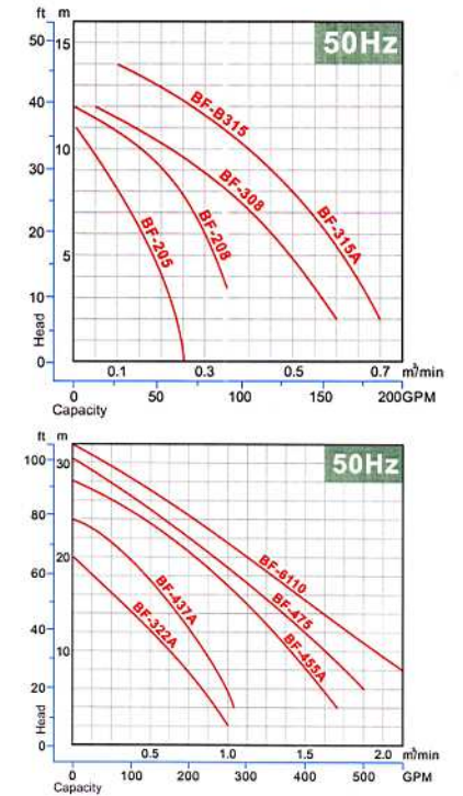
性能曲線圖
